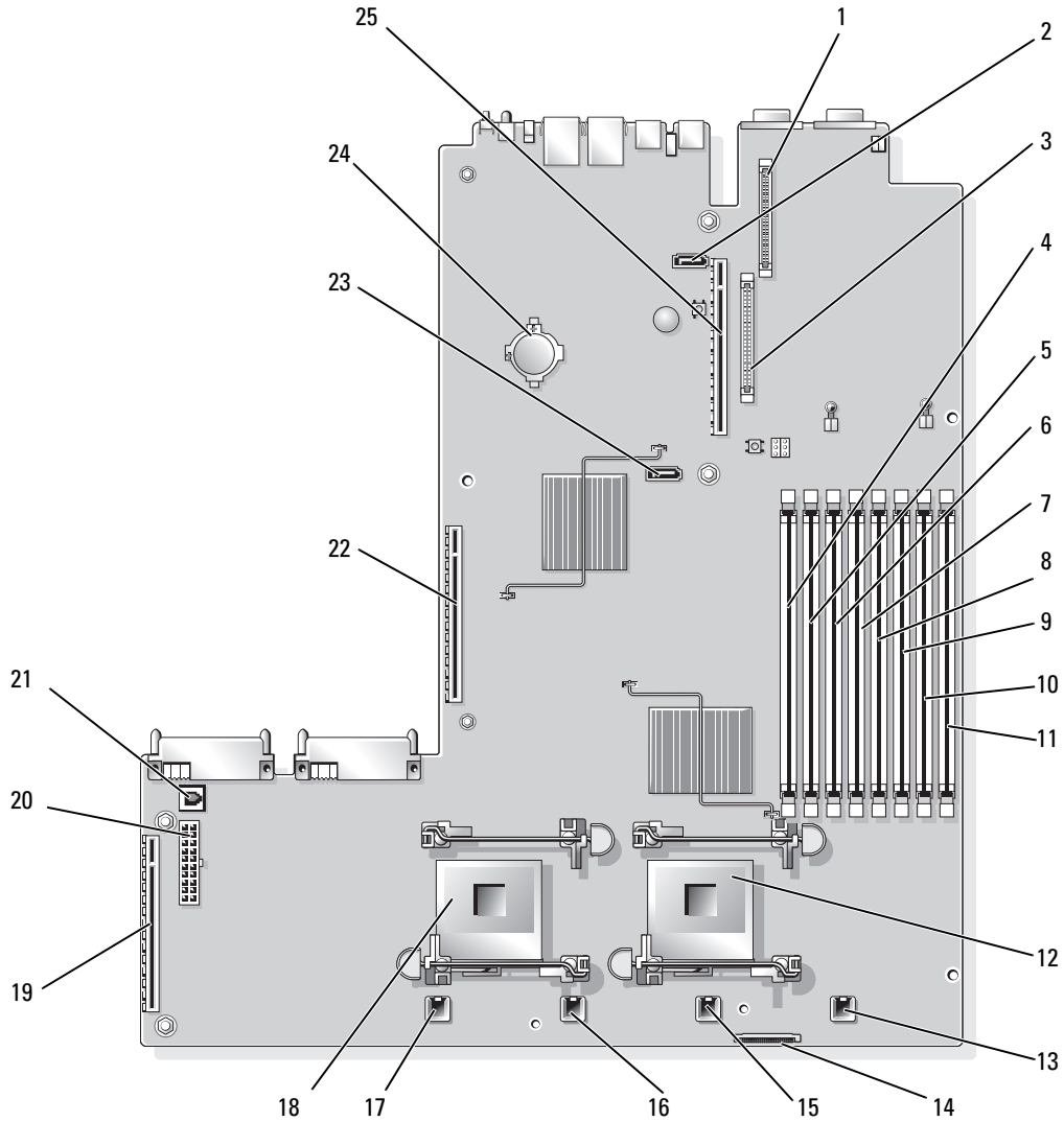
그림 6-2. 시스템 보드 커넥터
