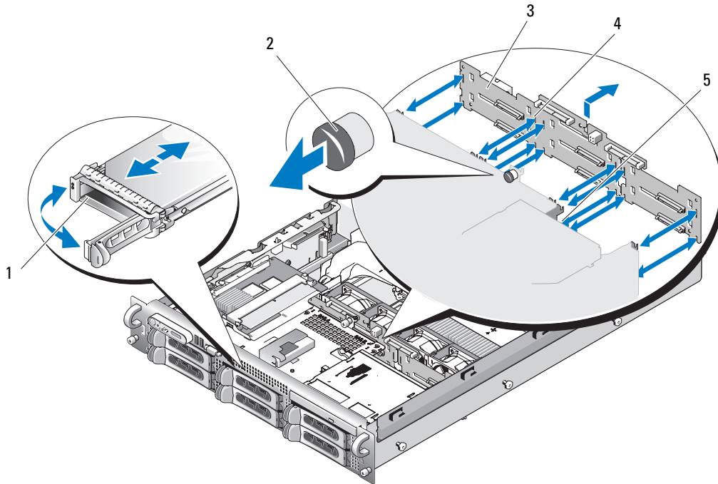
그림 3-34. SAS 후면판 board 분리
