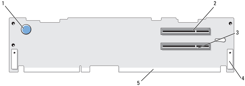
그림 6-7. 선택 사양인 PCIe 좌측 확장 카드 라이저 보드 구성요소
