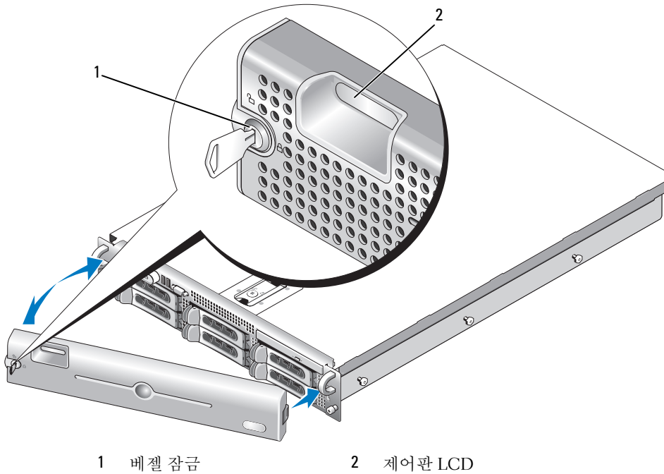
그림 3-2. 전면 베젤 분리
