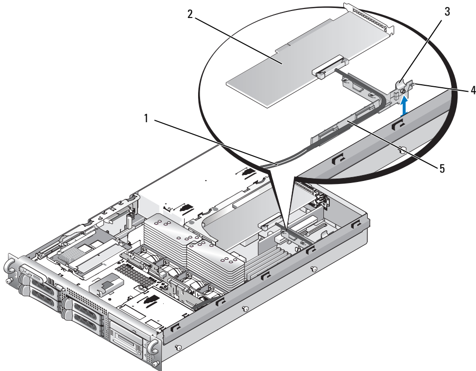
그림 3-26. 테이프 드라이브 케이블 고정 브래킷 설치 및 분리
