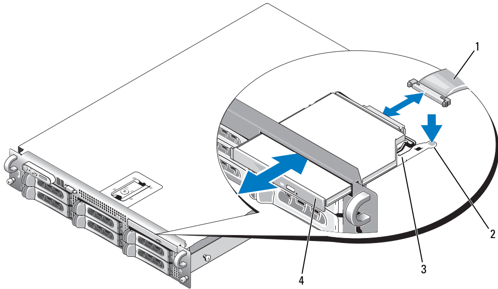
그림 3-21. 광학 드라이브 트레이 분리 및 설치
