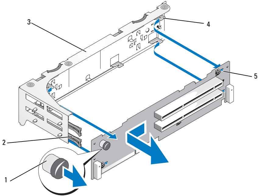
그림 3-31. 좌측 라이저 보드 장착
