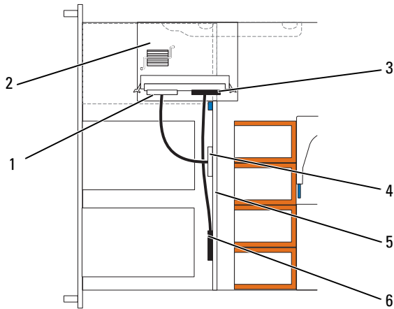
그림 3-14. 3.5 인치 x6 후면판에 SAS RAID 컨트롤러 보조 카드 케이블 연결
