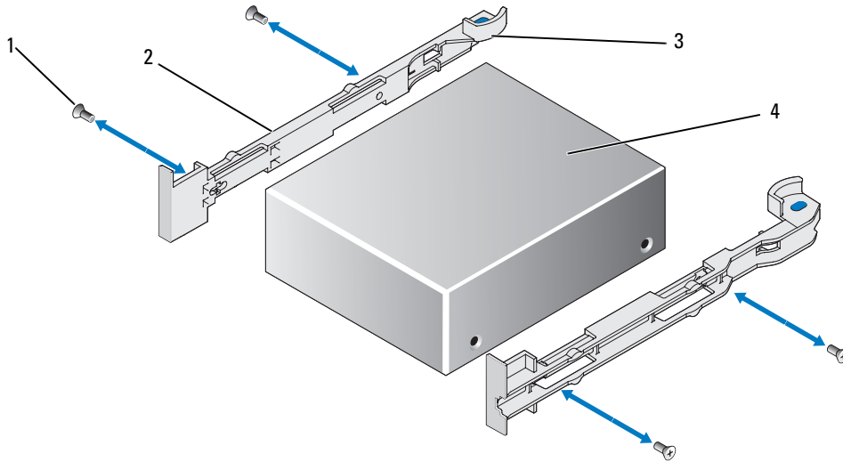
그림 3-25. 내장형 SCSI 테이프 드라이브 분리 및 설치
