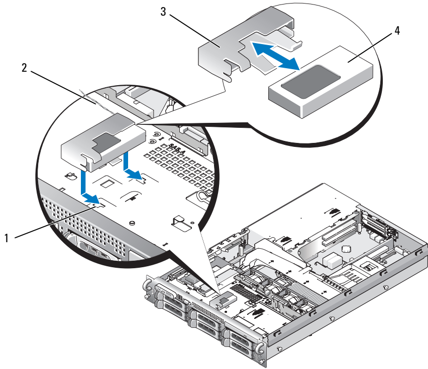
그림 3-17. RAID 전지 설치
