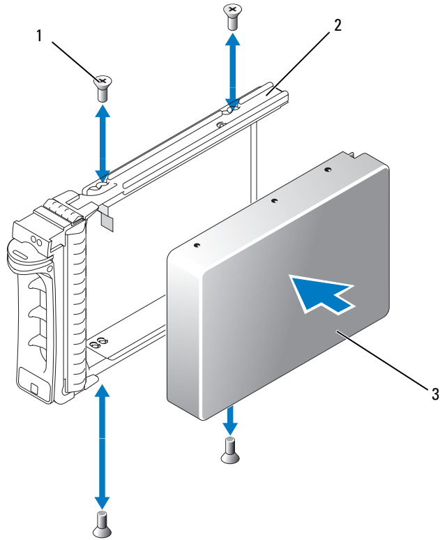
그림 3-6. SATA 드라이브 캐리어에 SATA 하드 드라이브 설치
