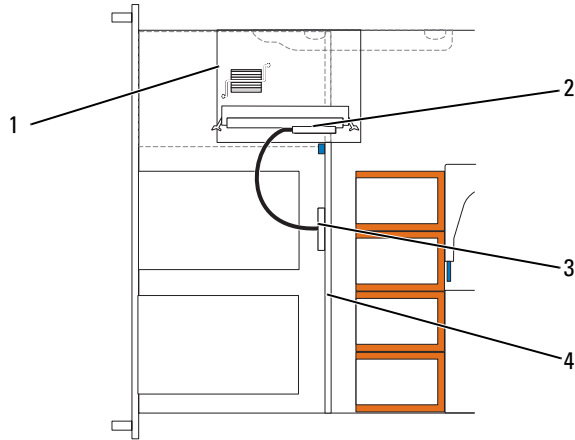
그림 3-13. 모든 후면판에 SAS 컨트롤러 보조 카드 케이블 연결
