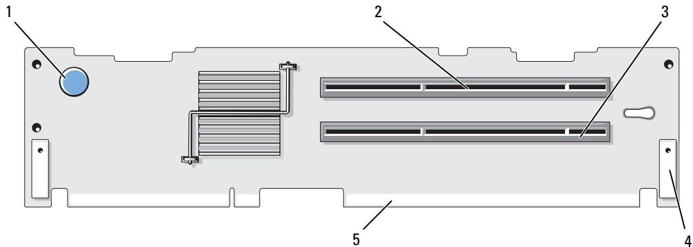
그림 6-8. 선택 사양인 PCI-X 좌측 확장 카드 라이저 보드 구성요소
