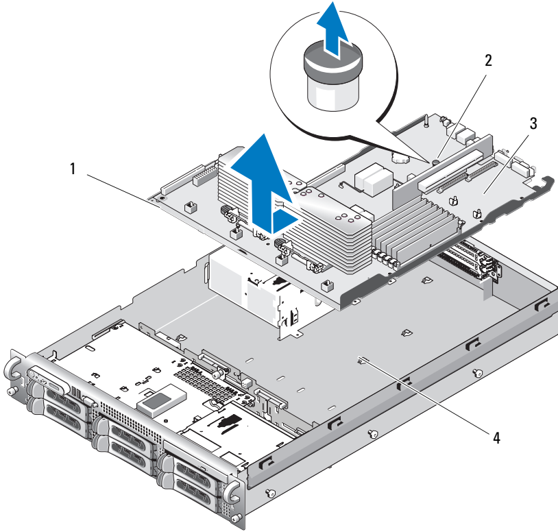
그림 3-36. 시스템 보드 분리
