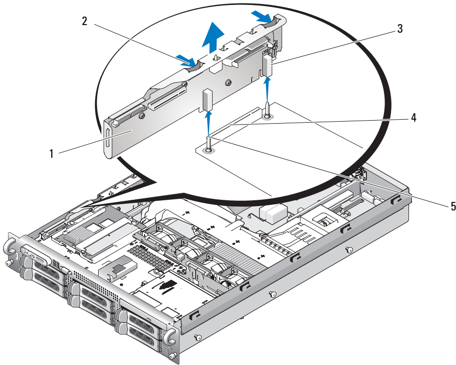
그림 3-33. 측면판 분리 및 설치
