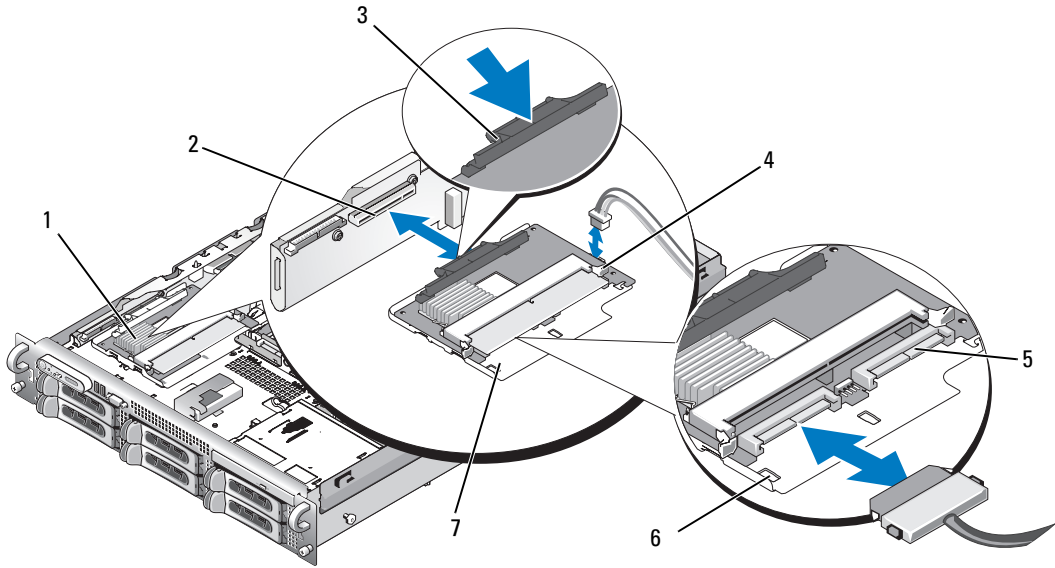
그림 3-12. SAS 컨트롤러 보조 카드 설치
