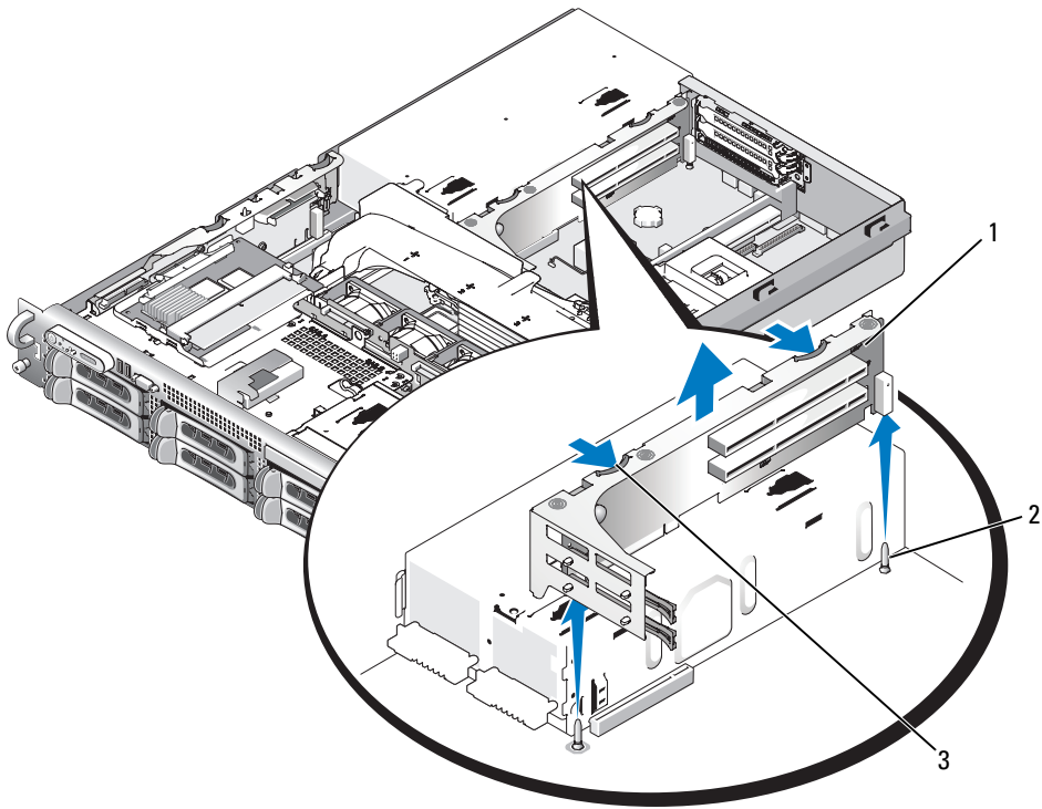
그림 3-19. 확장 카드 케이지 설치 및 분리
