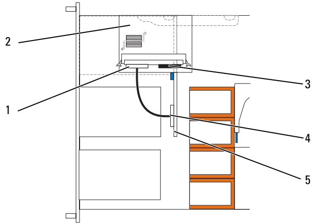
그림 3-15. 3.5 인치 x4 후면판에 SAS RAID 컨트롤러 보조 카드 케이블 연결
