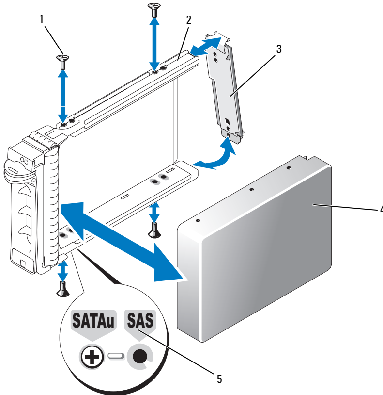
그림 3-7. SATAu 드라이브 캐리어에 SATA 하드 드라이브 및 접속기 카드 설치
