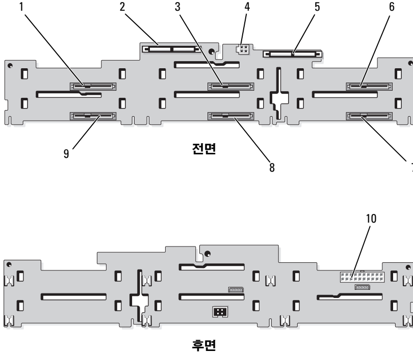
그림 6-3. SAS 후면판 보드 구성요소 : 3.5 인치 x6 옵션
