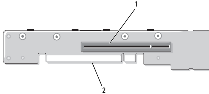
그림 6-9. 선택 사양인 PCIe 확장 카드 중앙 라이저 보드 구성요소
