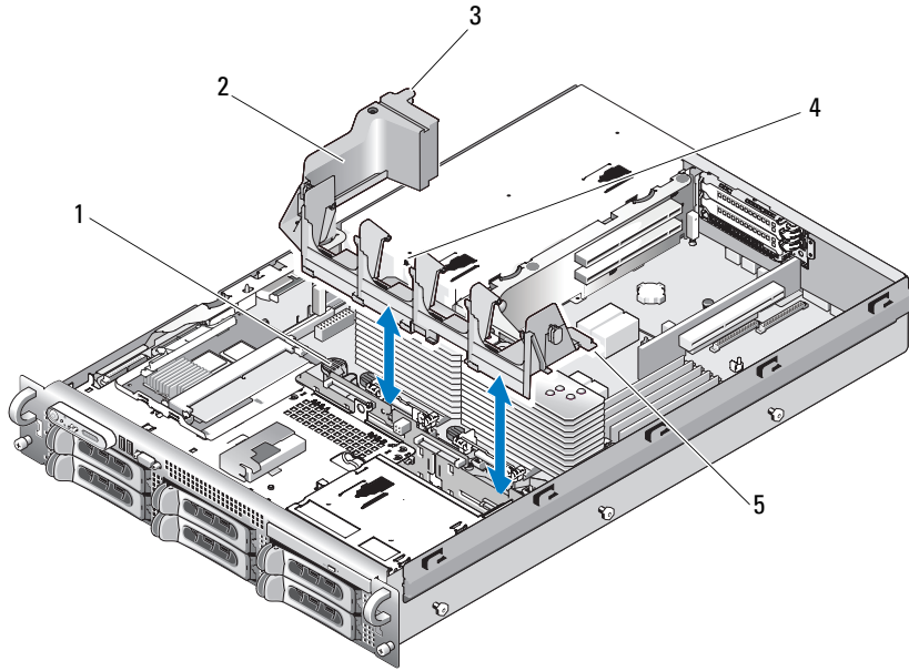
그림 3-11. 팬 브래킷 분리 및 설치
