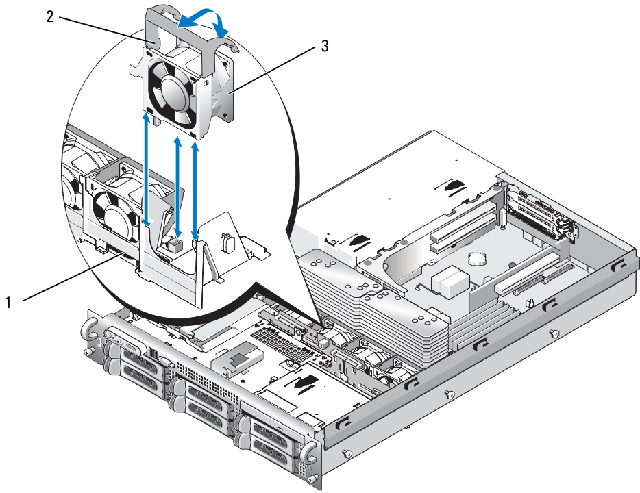
그림 3-9. 냉각팬 분리 및 설치
