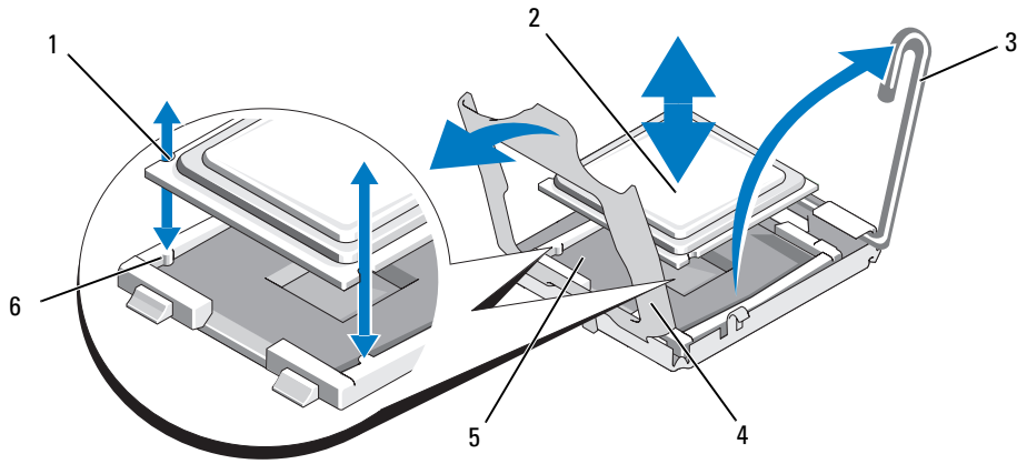
그림 3-29. 프로세서 설치 및 분리
