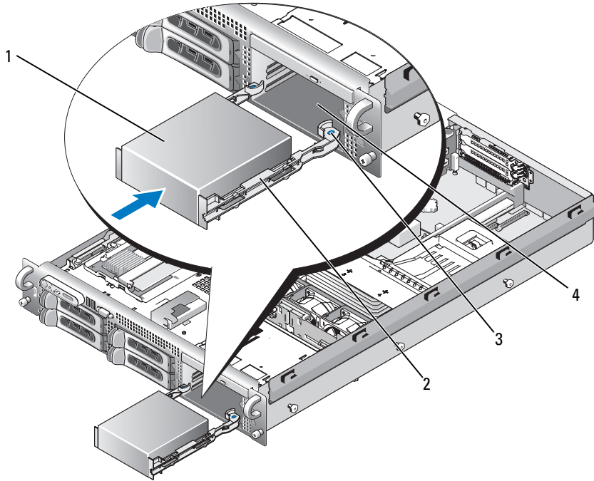
그림 3-24. 테이프 드라이브 캐리어 분리 및 설치
