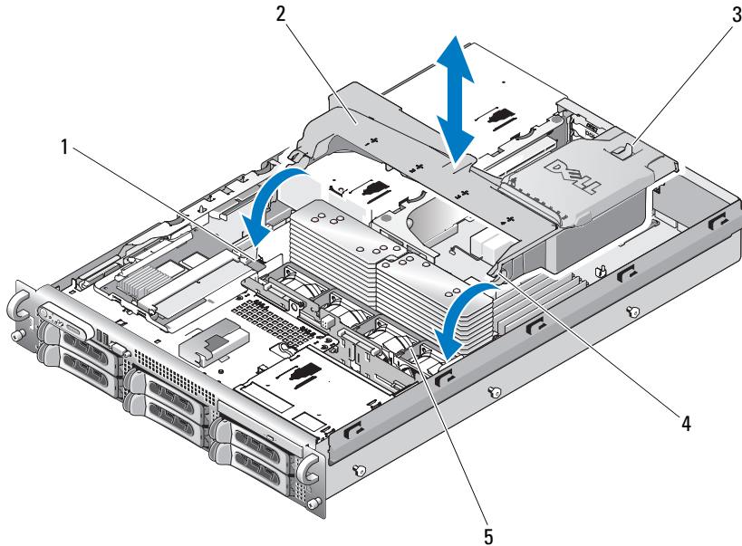
그림 3-10. 냉각 덮개 분리 및 설치
