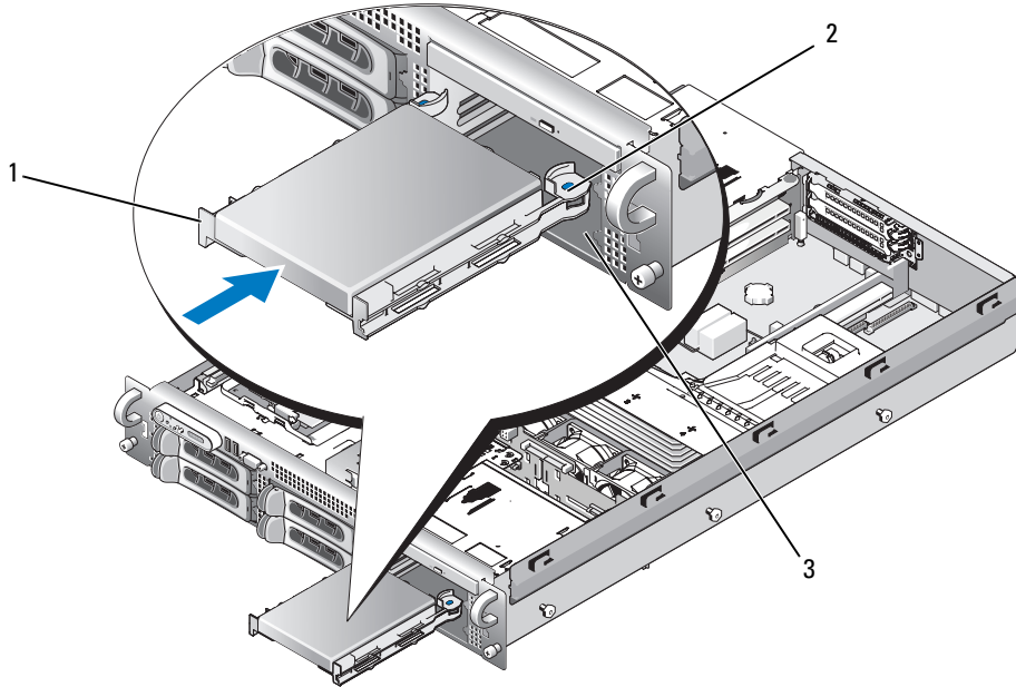
그림 3-22. 시스템에 디스켓 드라이브 설치 및 분리
