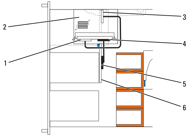
그림 3-16. 2.5 인치 x8 후면판에 SAS RAID 컨트롤러 보조 카드 케이블 연결
