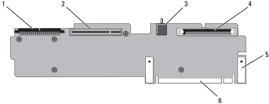
그림 6-6. 측면판 보드 커넥터
