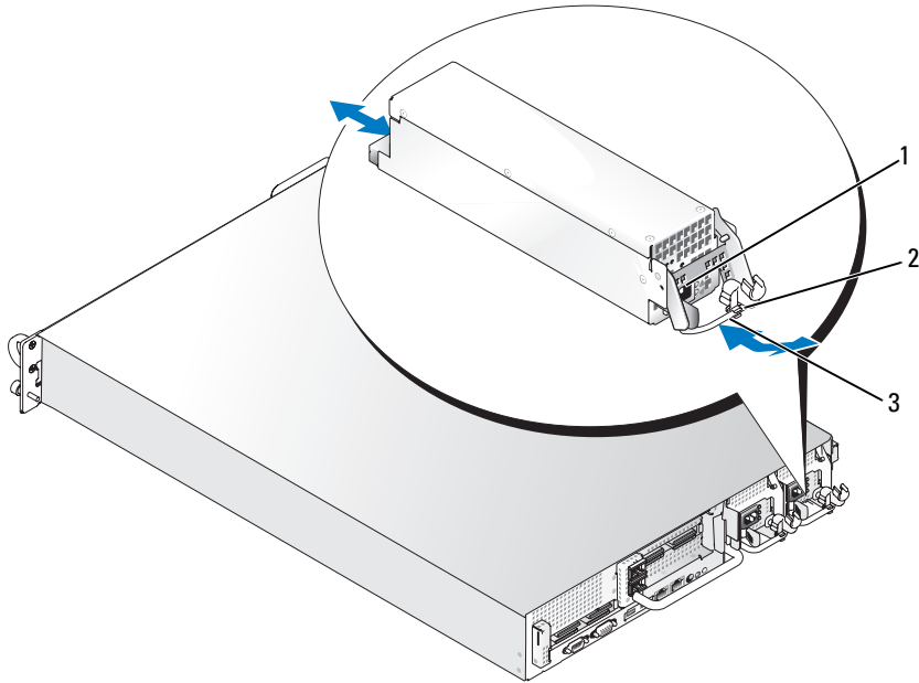
그림 3-8. 전원 공급 장치 분리 및 설치
