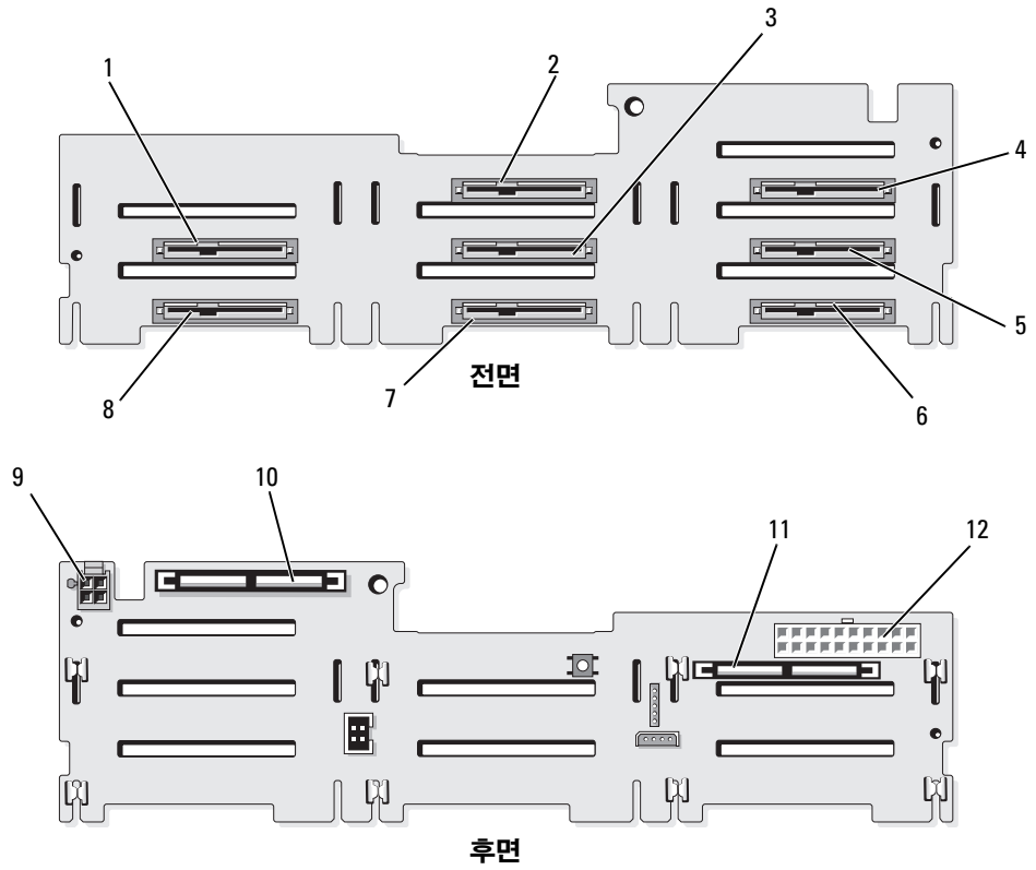
그림 6-5. SAS 후면판 보드 구성요소 : 2.5 인치 x8 옵션
