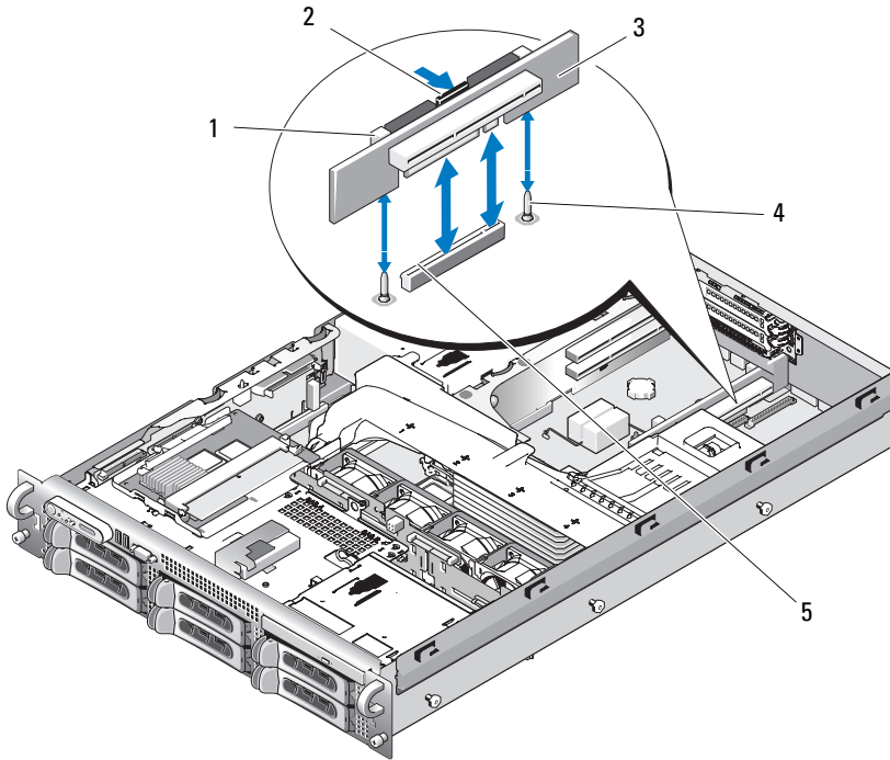
그림 3-32. 중앙 라이저 보드 장착
