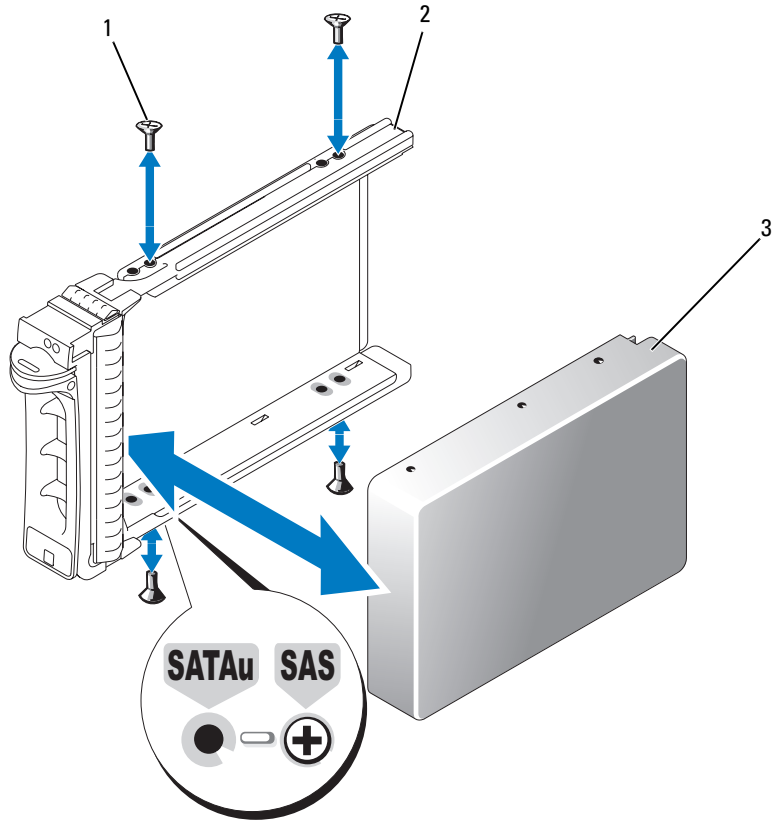
그림 3-5. SATAu 드라이브 캐리어에 SAS 하드 드라이브 설치
