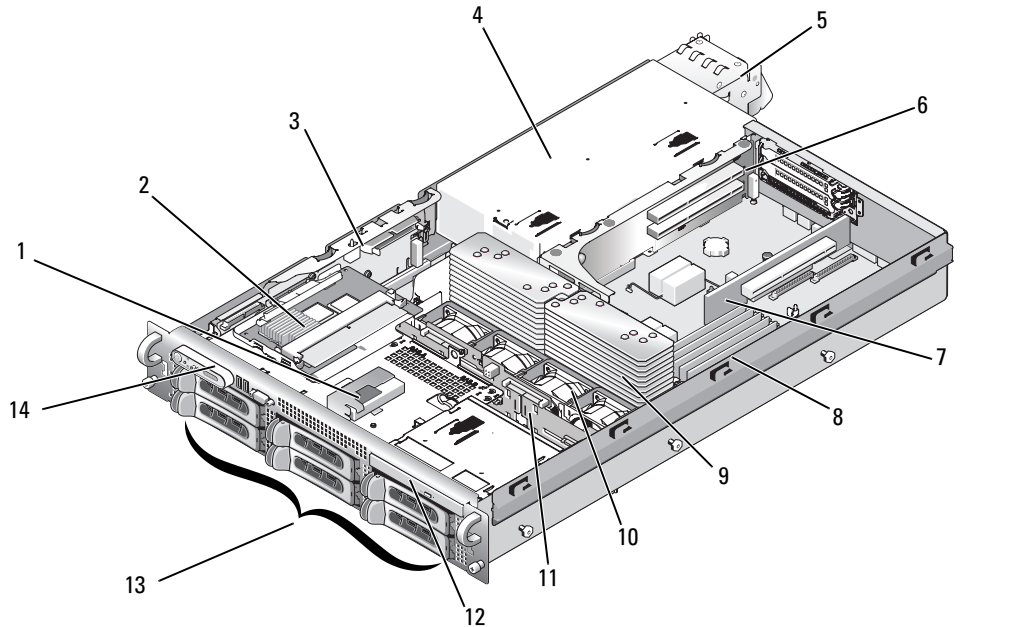
그림 3-1. 시스템 내부
