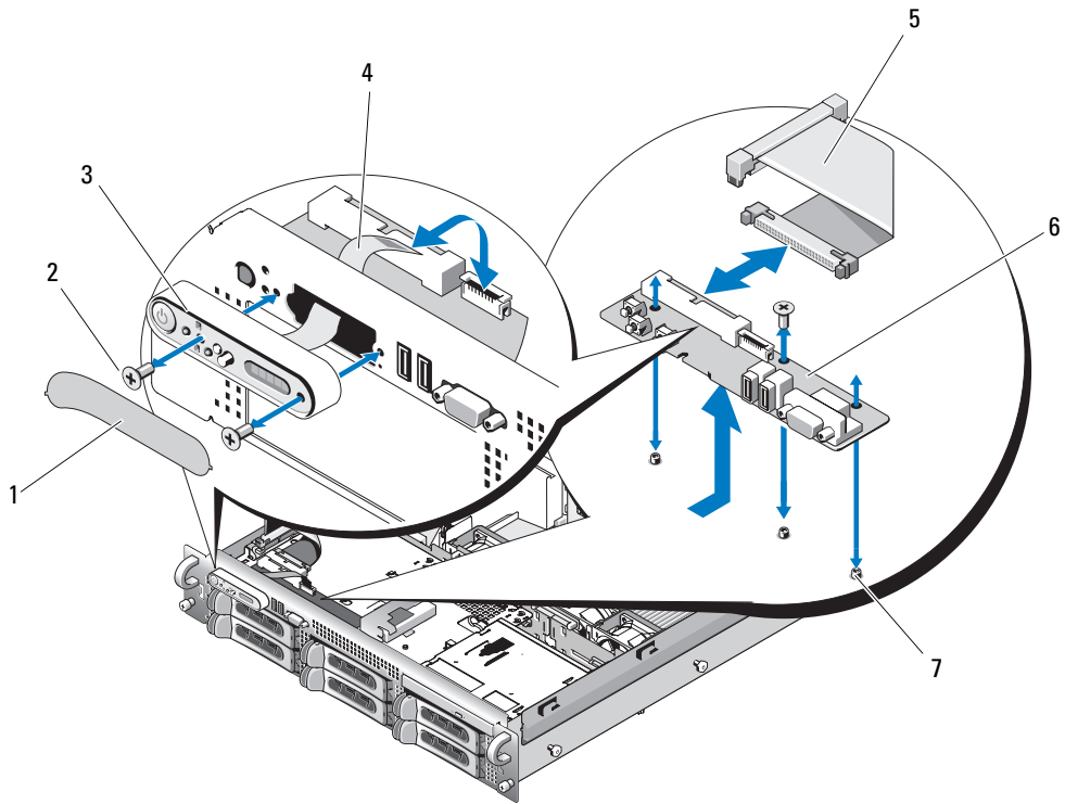
그림 3-35. 제어판 분리
