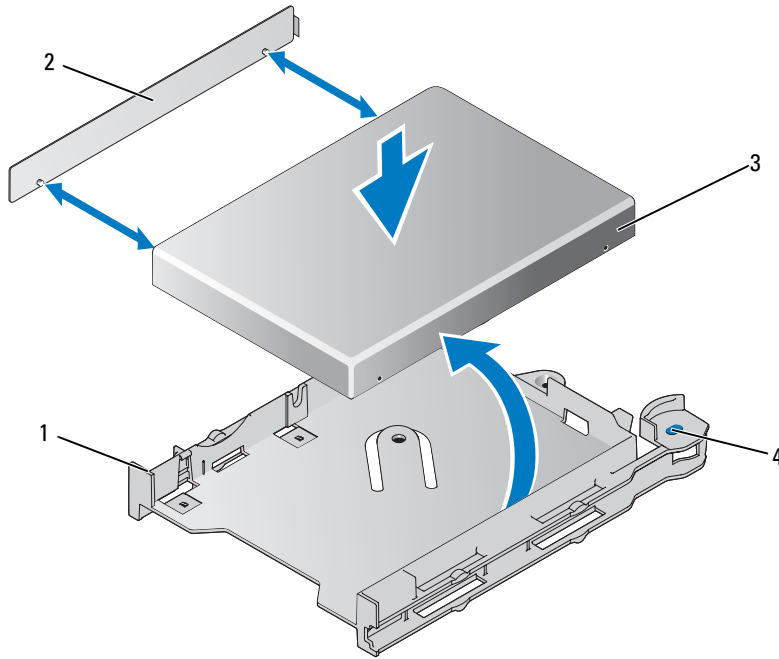
그림 3-23. 드라이브 캐리어에 디스켓 드라이브 설치 및 드라이브 캐리어에서 디스켓 드라이브 분리
