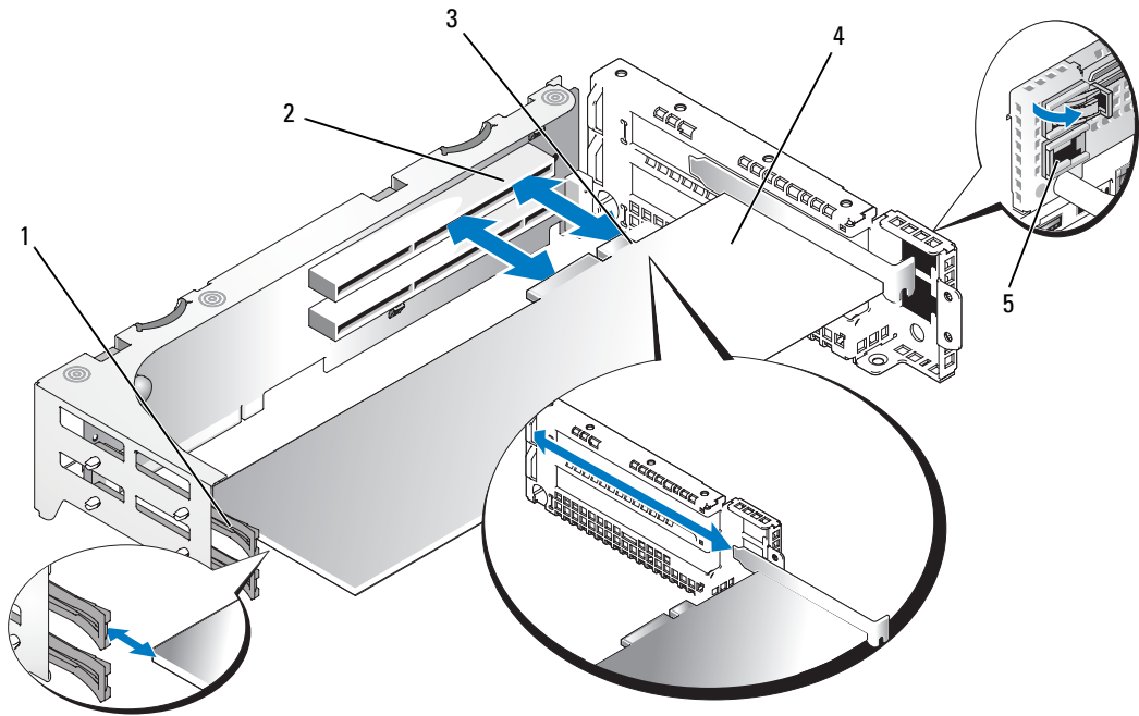
그림 3-18. 확장 카드 설치
