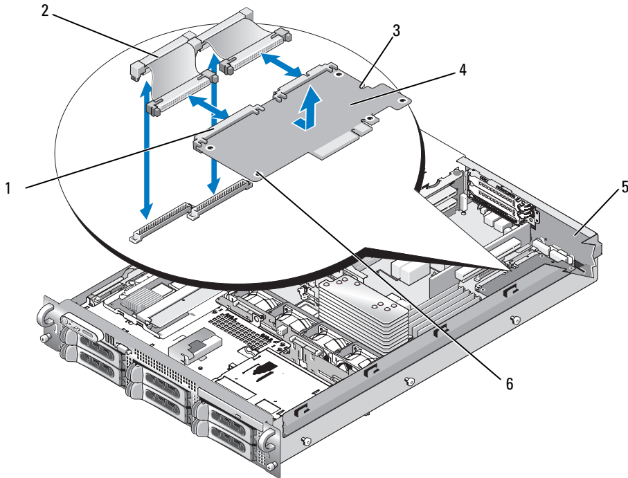
그림 3-20. RAC 카드 설치
