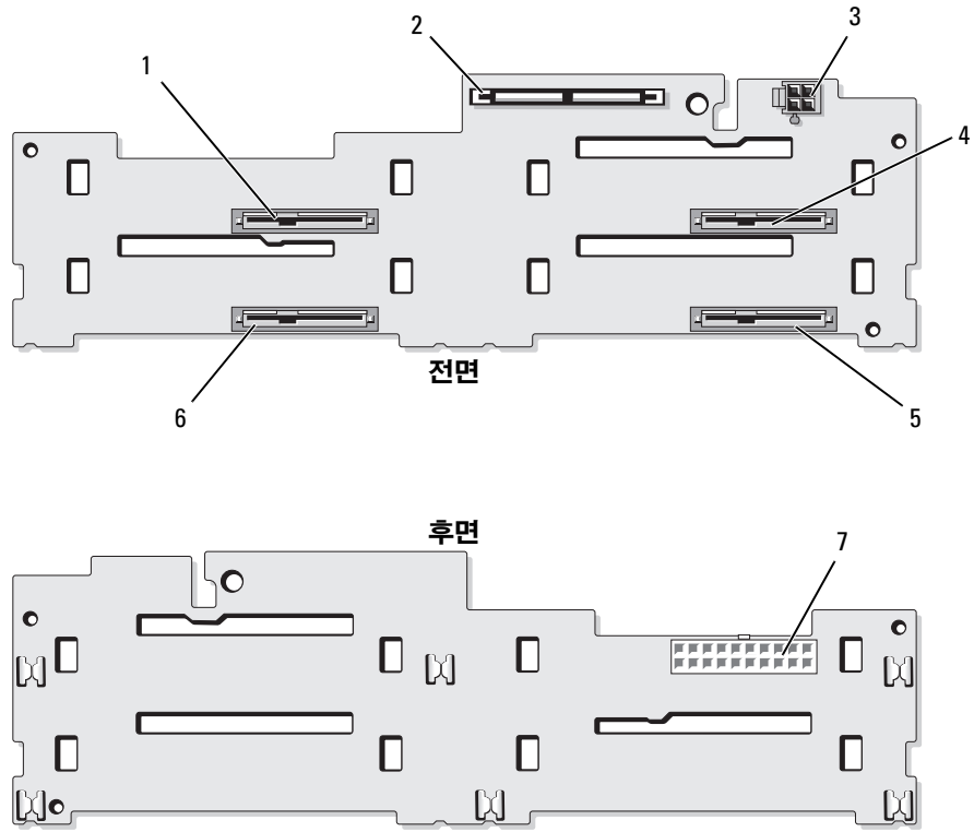
그림 6-4. SAS 후면판 보드 구성요소 : 3.5 인치 x4 옵션
